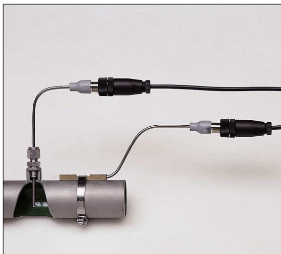
Esempi di installazione con accessori
