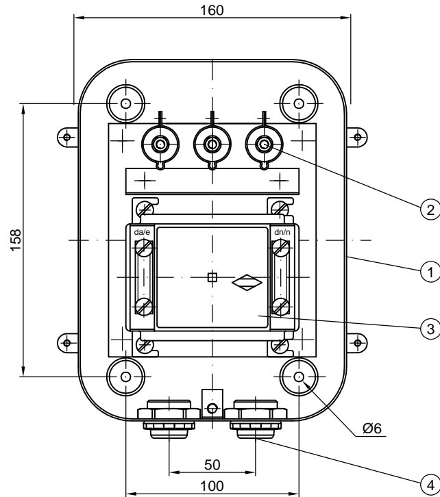
Ansicht ohne Deckel view without cover
